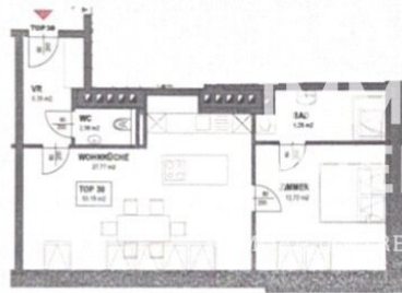
1. Dachgeschoß
