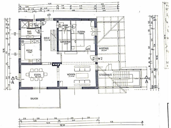
OBERGESCHOSS
