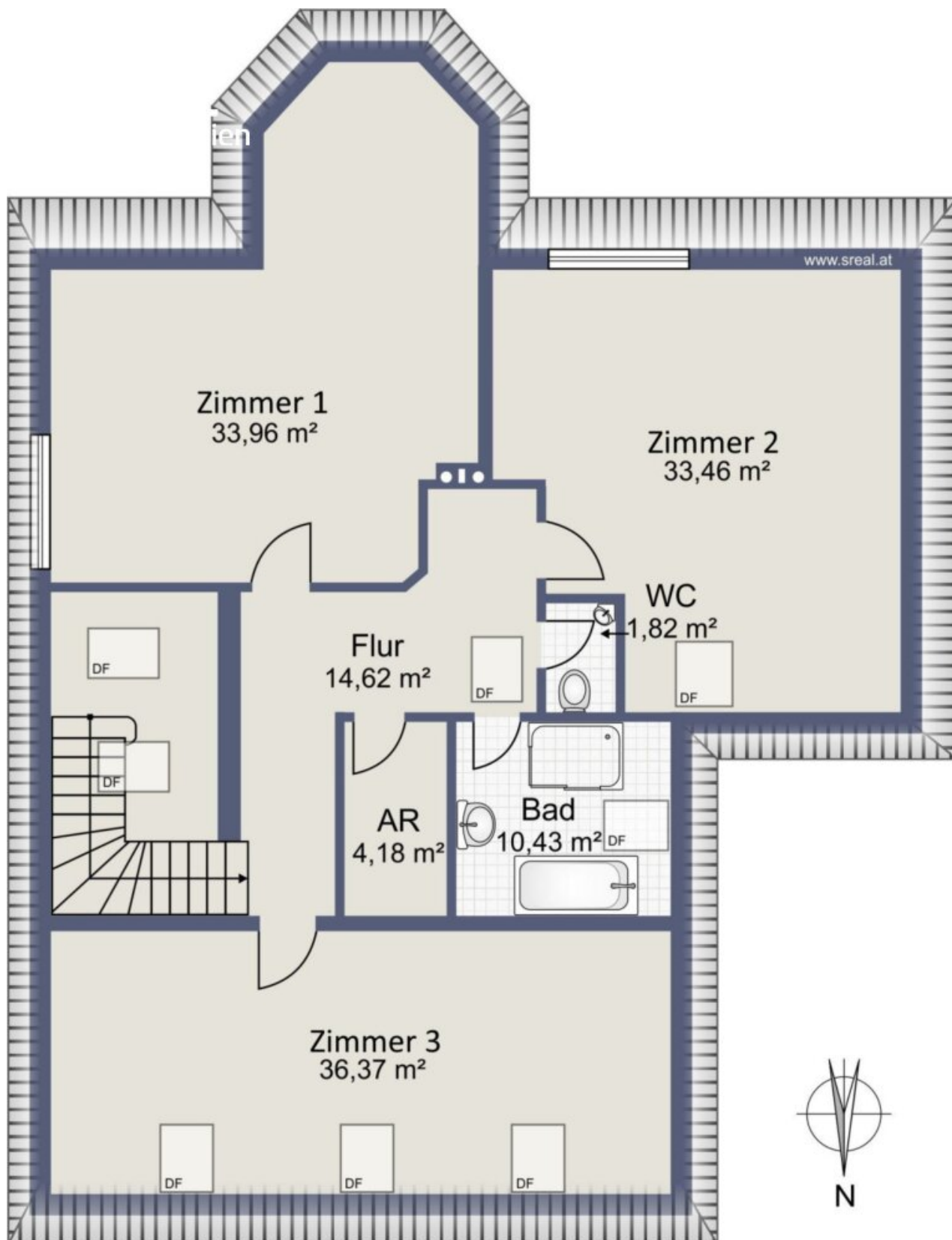
Planskizze Obergeschoss
