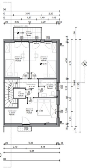
OBERGESCHOSS
