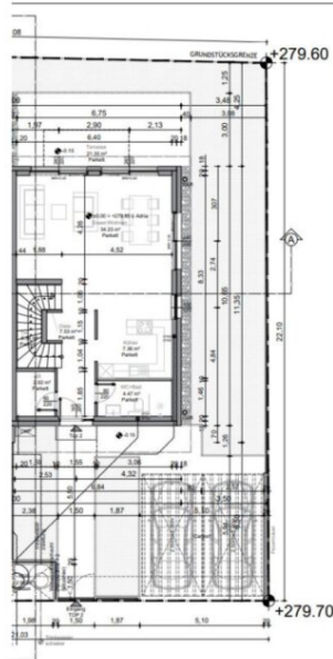
ERDGESCHOSS
