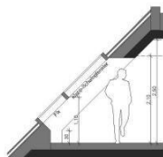
Schnitt 1
