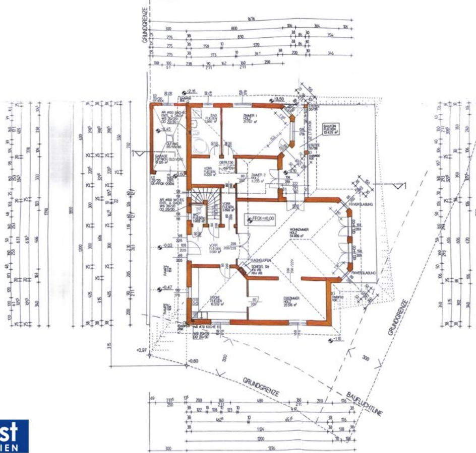
ERDGESCHOSS
