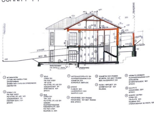
SCHNITT 1-1
