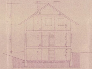
Schnitt AD
