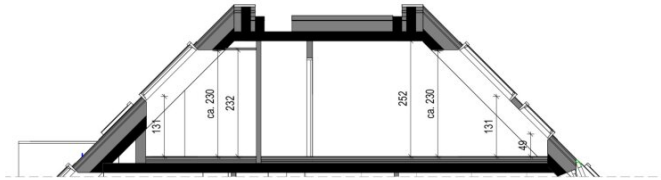
Schnitt 43.B
