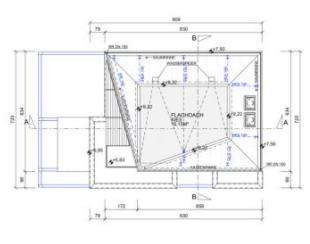
DACHDRAUFSICHT
