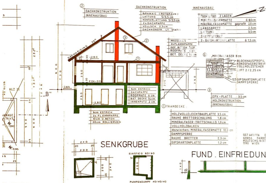
SCHNITT „A“-„B“
