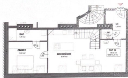
1. Dachgeschoß
