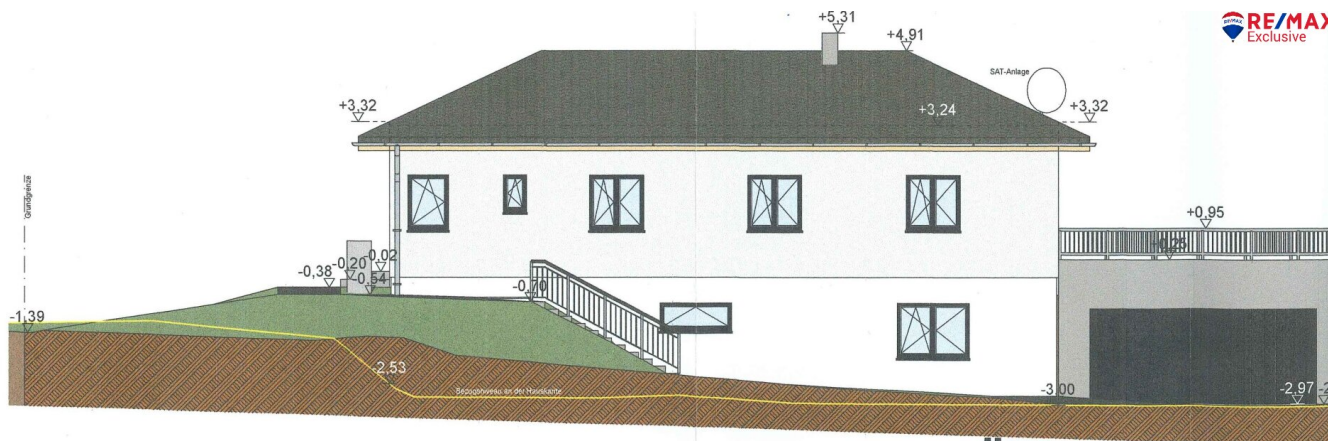
ANSICHT SÜD
