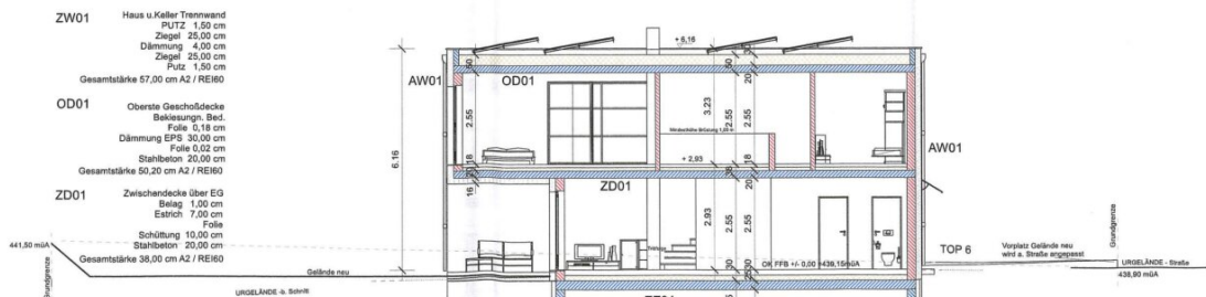
SCHNITT B-B
