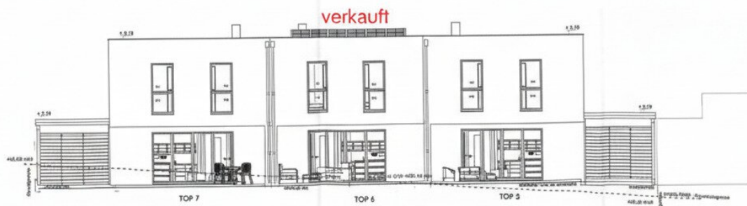
SÜDOSTANSICHT
