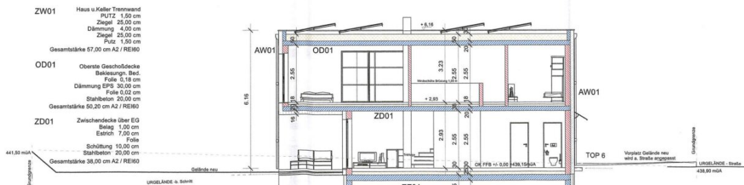
SCHNITT B-B
