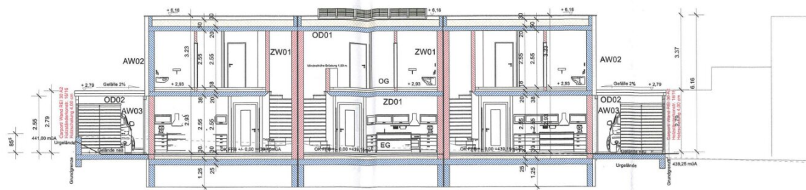
SCHNITT A-A
