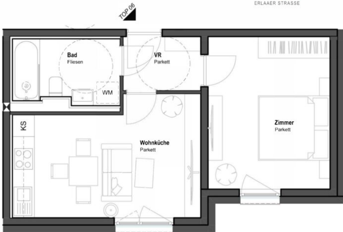
Grundriss 1:50
