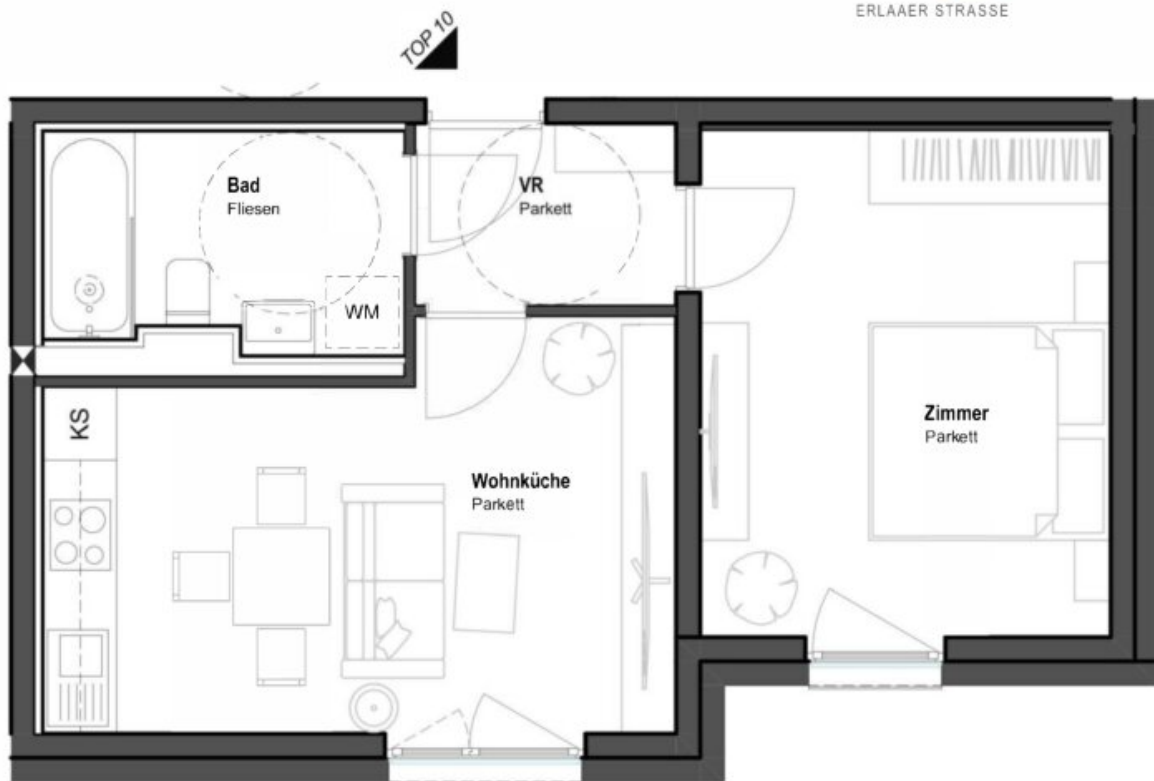
Grundriss 1:50
