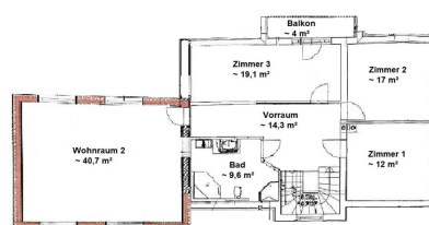
Obergeschoss-Skizze
