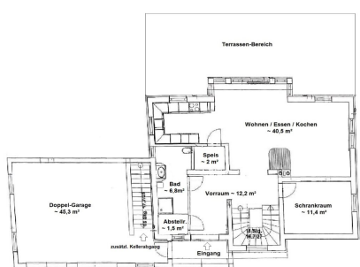
Erdgeschoss-Skizze
