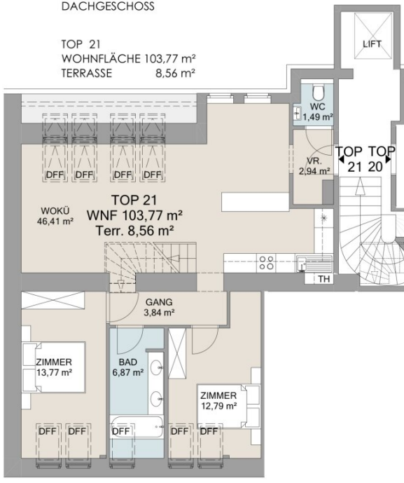
GRUNDRISS 1/100
