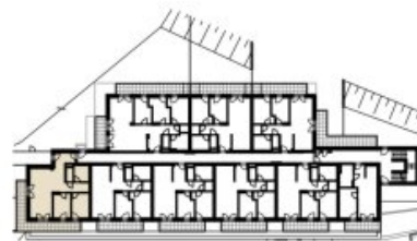
GRUNDRISS BK 03
