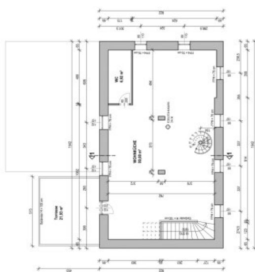
2. OBERGESCHOSS
