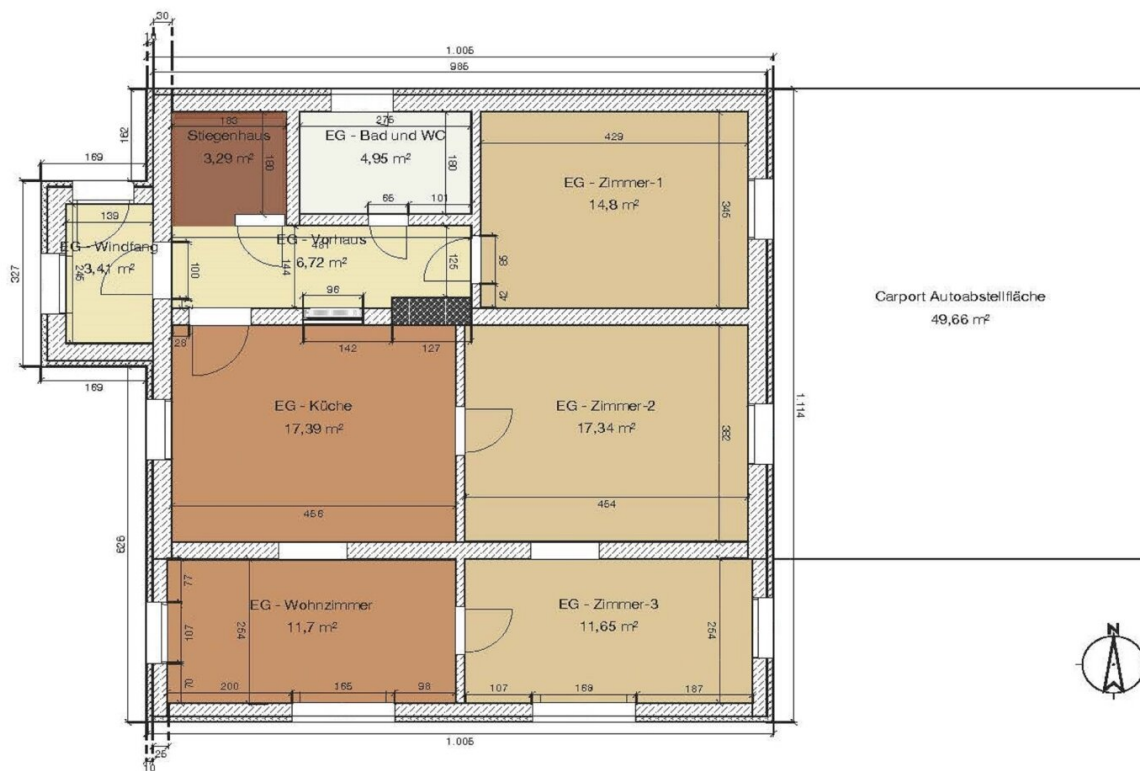
Grundriss-Skizze EG
