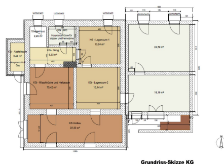
Grundriss-Skizze KG
