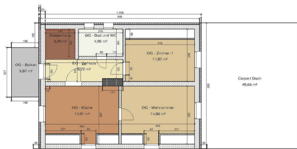
Grundriss-Skizze OG
