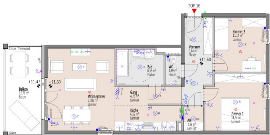
Übersicht 4. Obergeschoss M=1 : 1250
