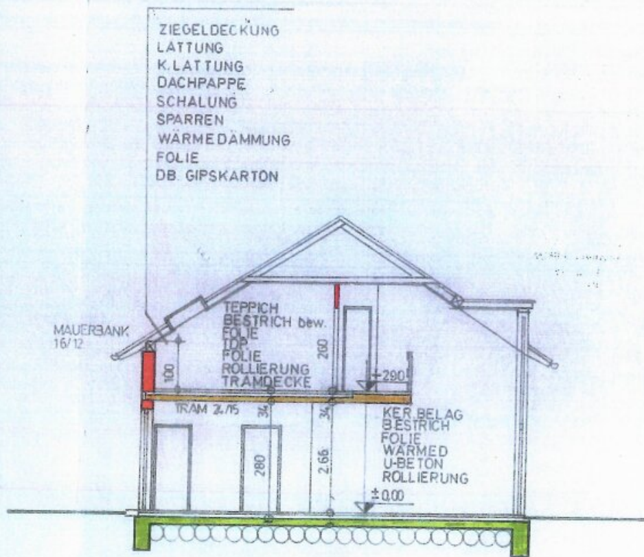
SCHNITT A-A
