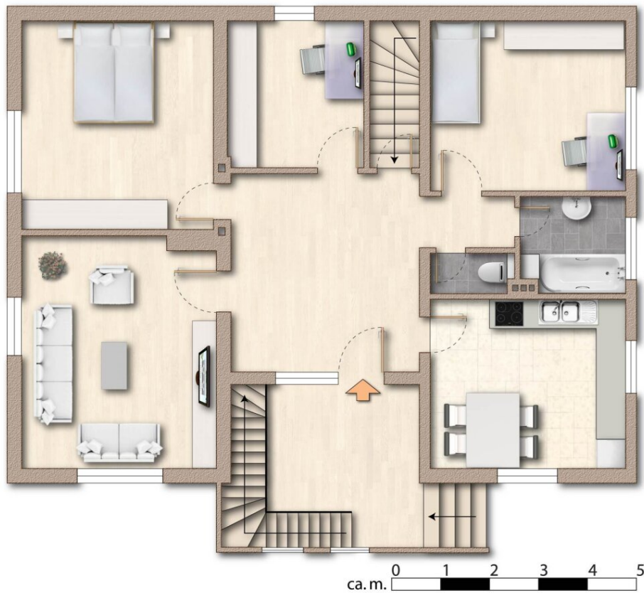
Grundriss Erdgeschoss möbliert
