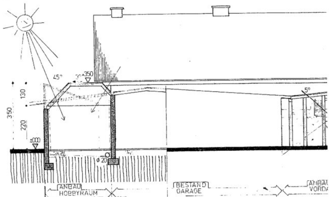
SCHNITT UND ANSICHT VON WESTEN
