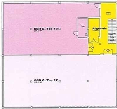
1. Obergeschoss M 1:100
