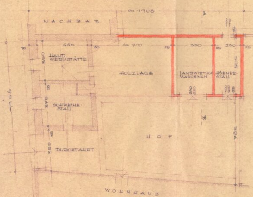
ERDGESCHOß
