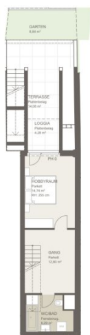
TÜR 11 Übersichtsplan Garten Maßstab 1:200
