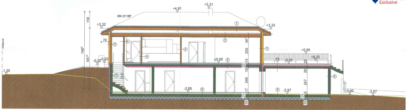
SCHNITT B-B
