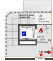
GRUNDRISSAUSSCHNITT 1.0G
