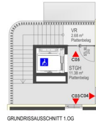
GRUNDRISSAUSSCHNITT 1.0G
