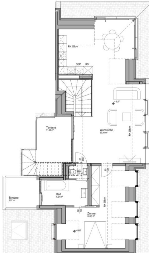
GR 2. Dachgeschoss
