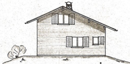
Vordansaicht
