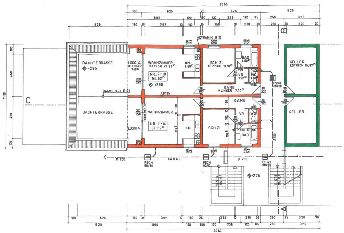
GRUNDRISS: REGELGESCHOSS
