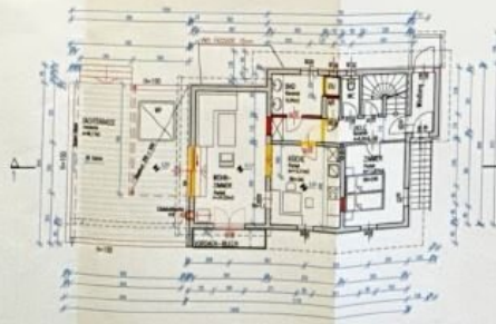
ERDGESCHOSS M 1/100
