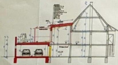
SCHNITT 1-1 M 1/100
