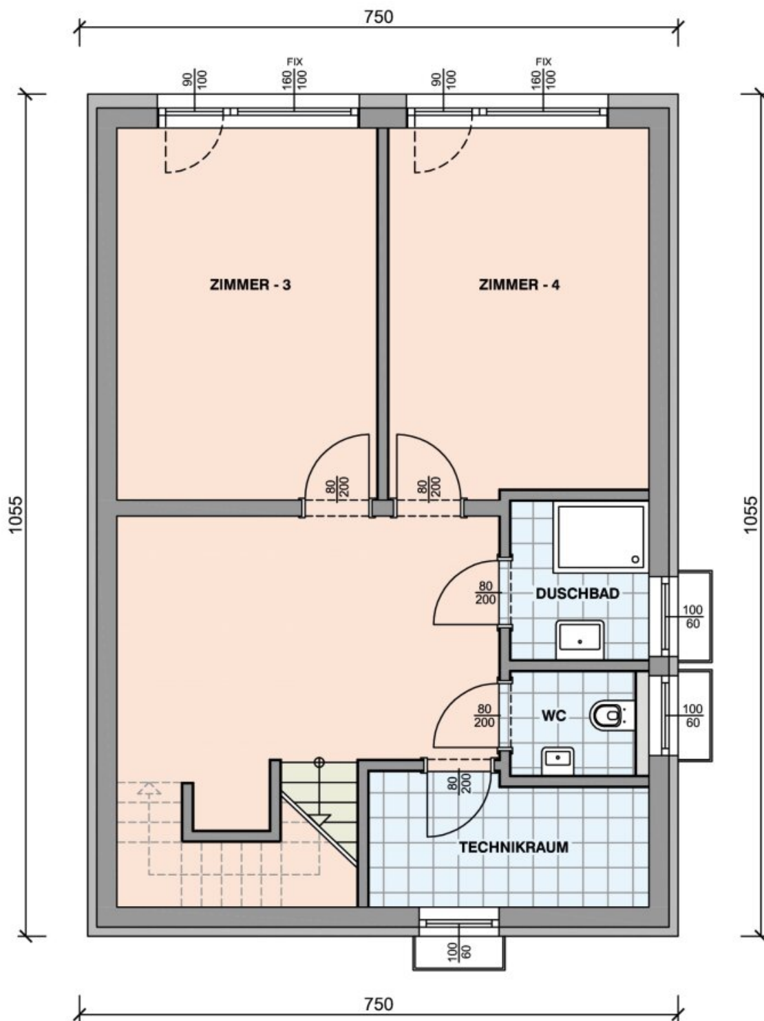
GRUNDRISS SOUTERRAIN
