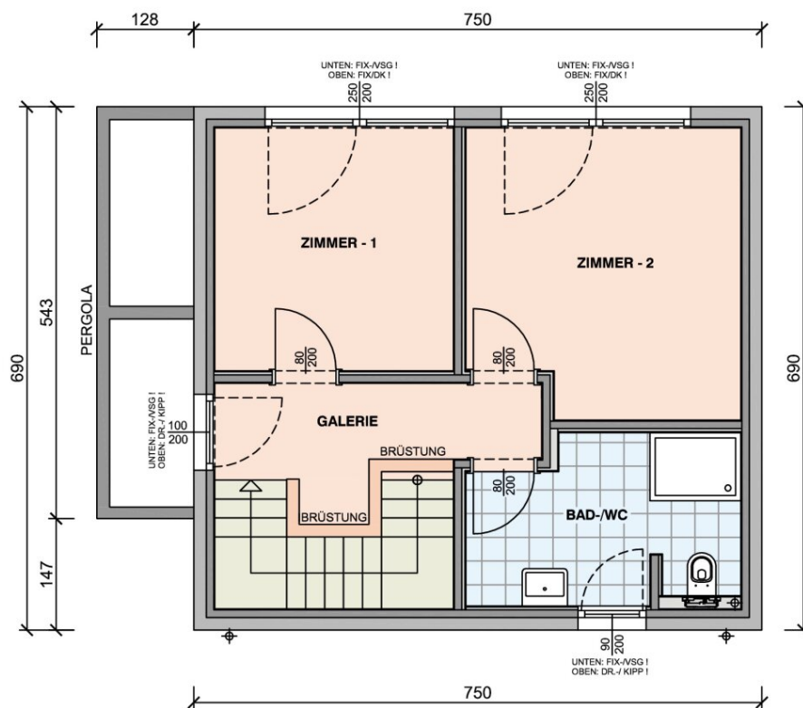
GRUNDRISS OBERGESCHOß
