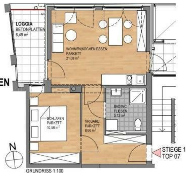
GRUNDRISS 1:100
