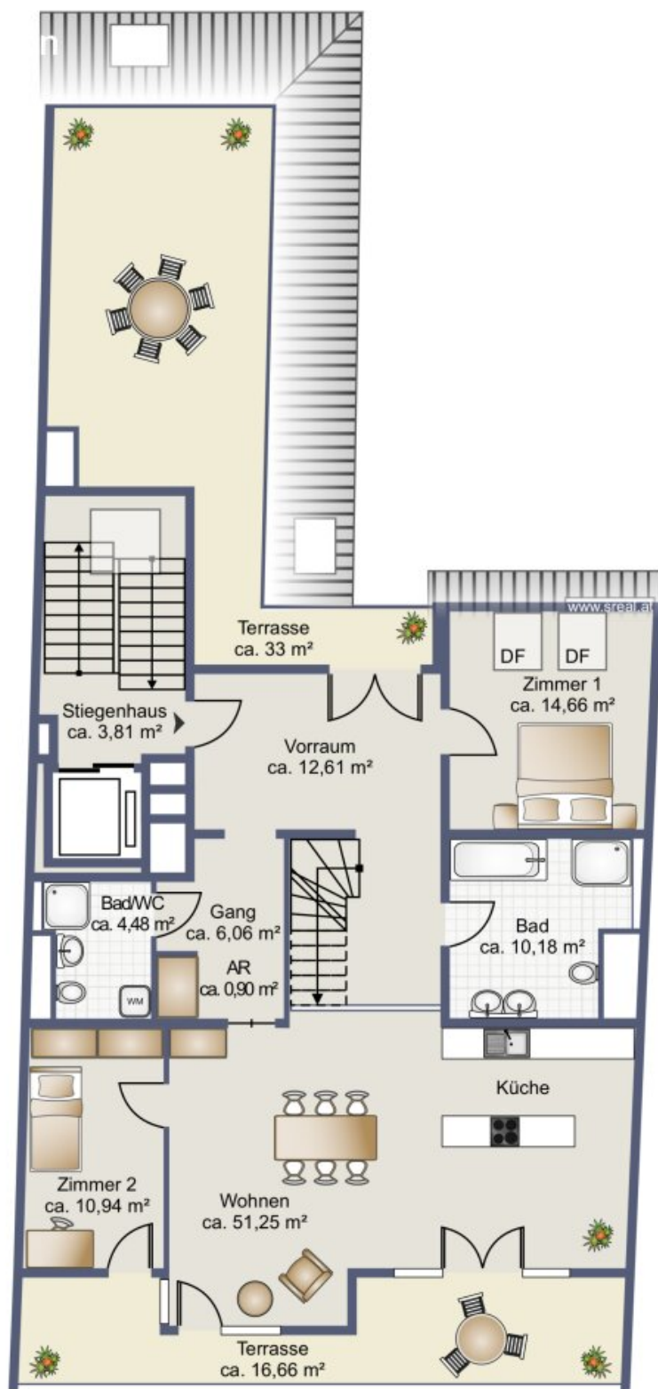
Skizze 1. Dachgeschoss
