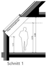
Schnitt 1
