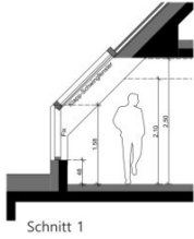
Schnitt 1
