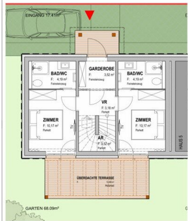
ERDGESCHOSS
