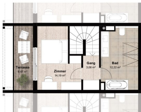
Dachgeschoss M 1:100
