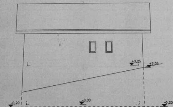
OST-ANSICHT 1:100
