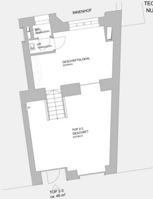
LAGEPLAN EG
