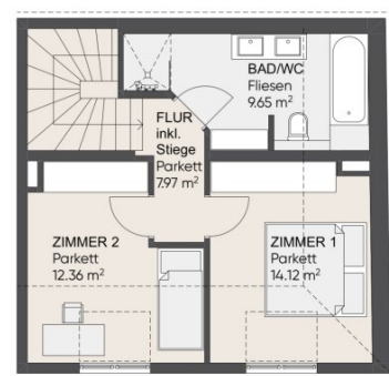
1. OG
