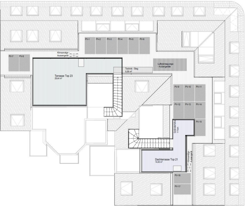
DACHDRAUFSICHT
