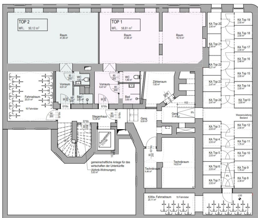
KELLERGECHOSS
