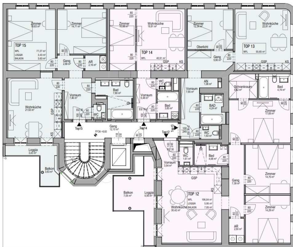
2. OBERGESCHOSS
