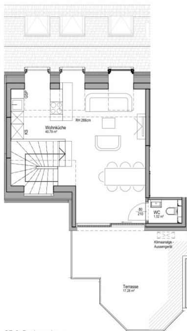
GR 2. Dachgeschoss
