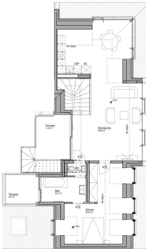
GR 2. Dachgeschoss
