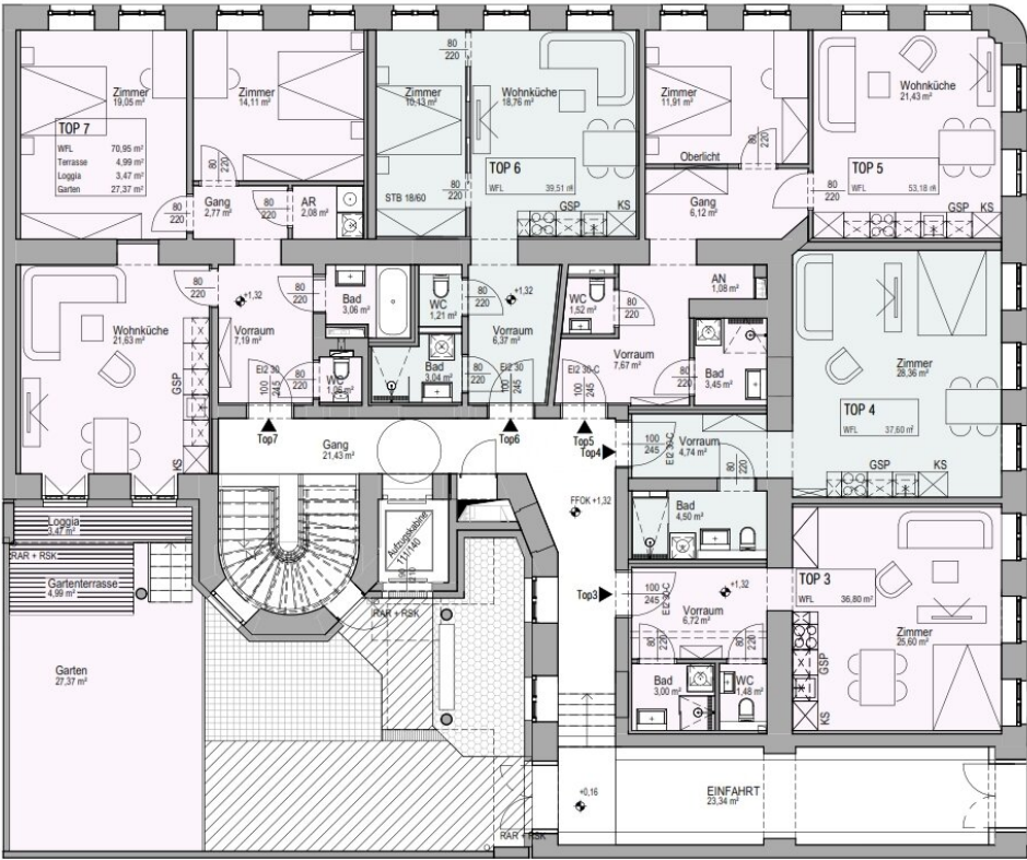
ERDGESCHOSS
