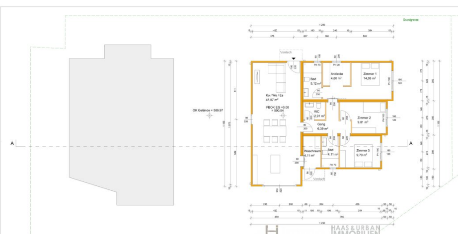
Grundriss Erdgeschoss M. 1:100 Austausch-Erreichung 24.10.2024
