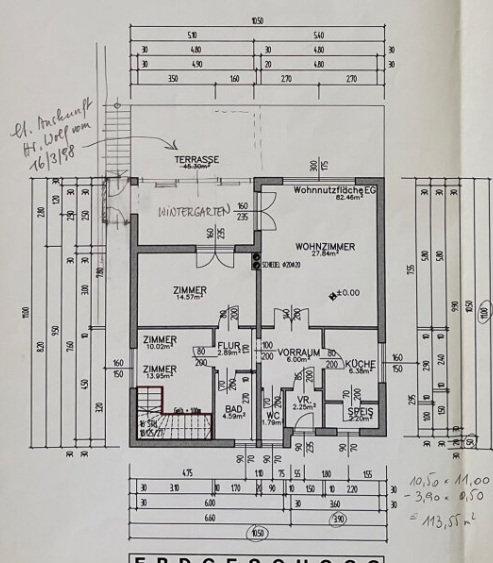
ERDGESCHOSS
