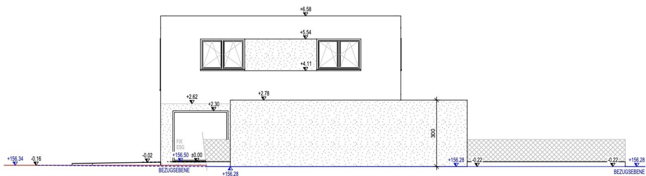
ANSICHT NORD-WEST
