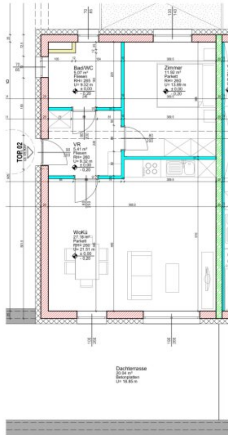
Planausschnitt 1.OBERGESCHOSS - Wohnung Planstand = Ausführungsplan M: 1:100
